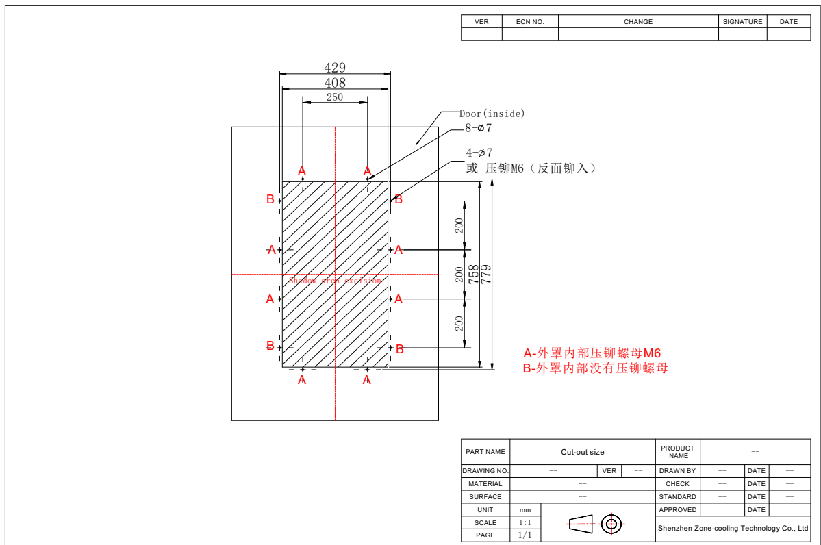
开孔尺寸图
