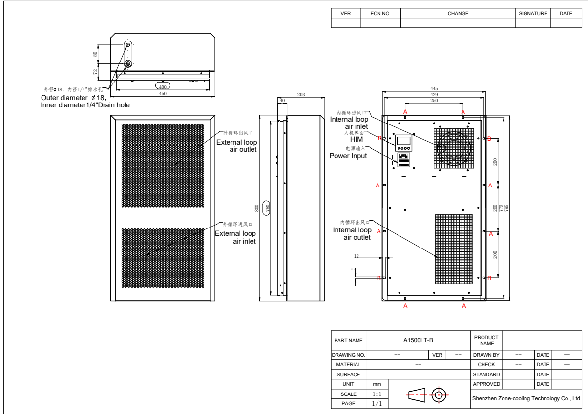
开孔尺寸图
