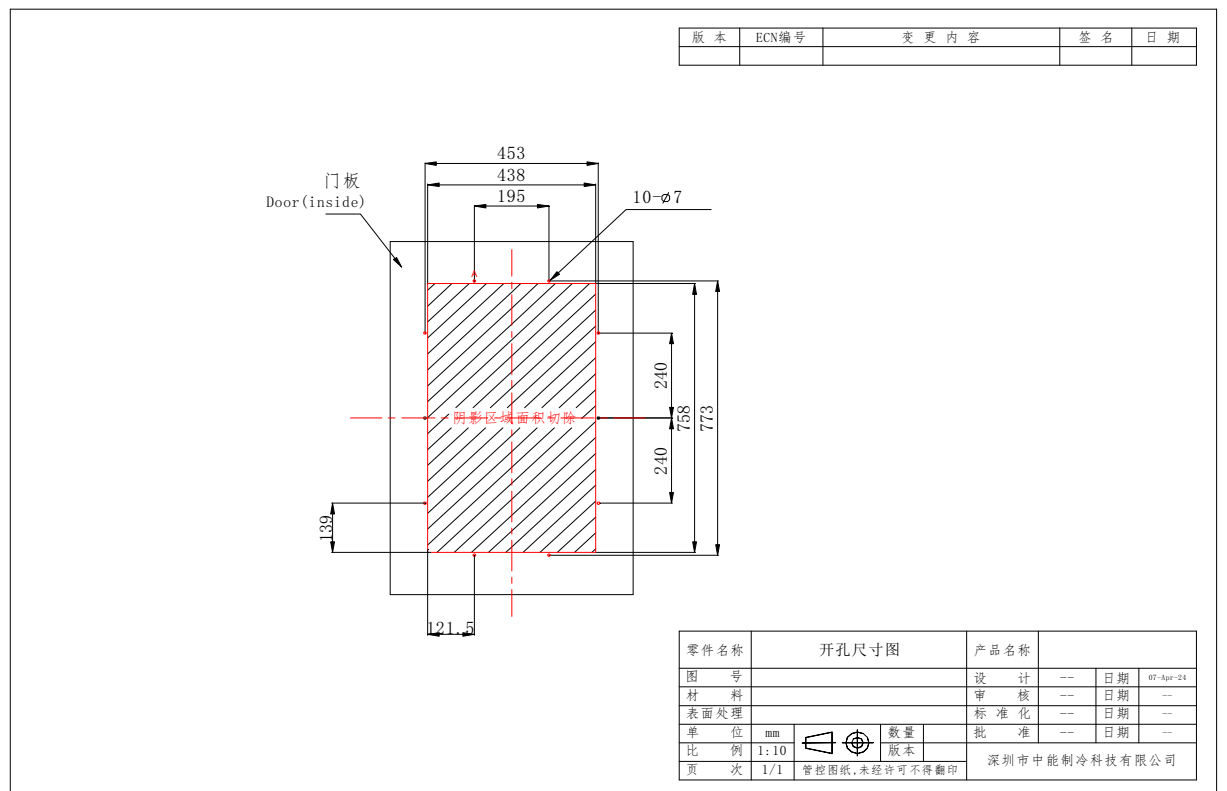
开孔尺寸图
